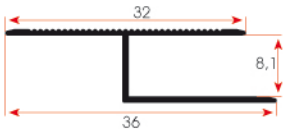
FSM 117 0,139 kg/m
