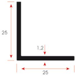
FSM 104 0,160 kg/m
