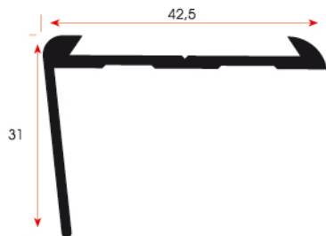
FSM 110 0,375 kg/m
