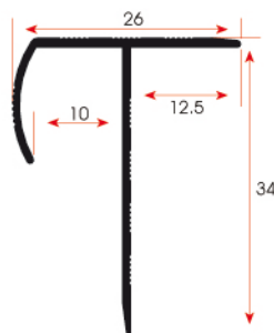
FSM 122 0,190 kg/m
