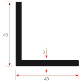
FSM 109 0,625 kg/m
