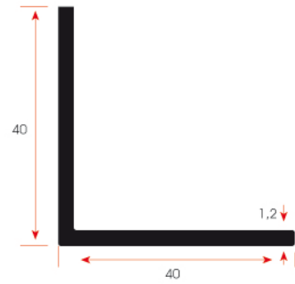
FSM 106 0,256 kg/m
