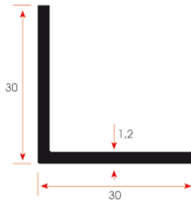
FSM 105 0,191 kg/m
