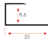
FSM 112 0,085 kg/m
