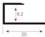
FSM 111 0,111 kg/m
