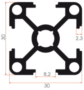
FSM 3002 0,818 kg/m
