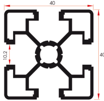
FSM 3004 1,059 kg/m
