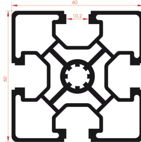
FSM 3003 2,619 kg/m
