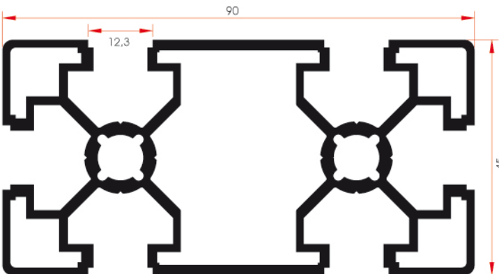
FSM 3007 2,480 kg/m
