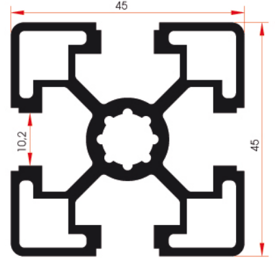
FSM 3006 1,587 kg/m
