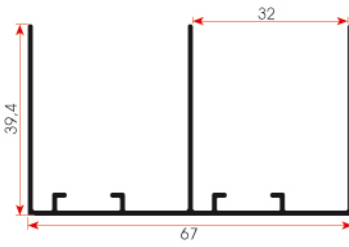
FSM 234 0,553 kg/m
