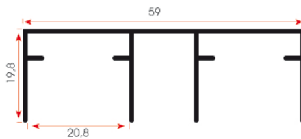
FSM 213 0,413 kg/m
