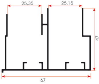
FSM 235 0,699 kg/m
