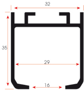
FSM 209 0,522 kg/m
