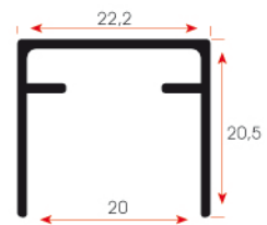
FSM 212 0,202 kg/m
