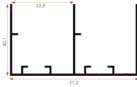
FSM 227 0,715 kg/m
