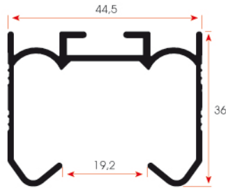
FSM 211 0,625 kg/m
