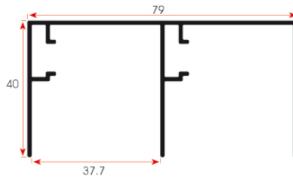
FSM 225 0,740 kg/m
