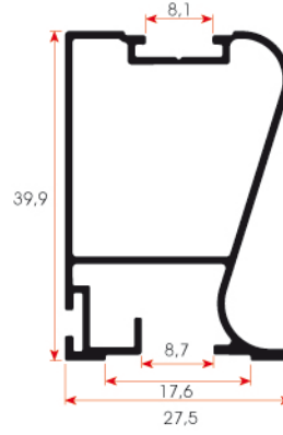
FSM 1034 0,425 kg/m
