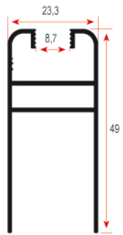
FSM 1005 0,469 kg/m
