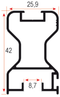
FSM 1001 0,480 kg/m
