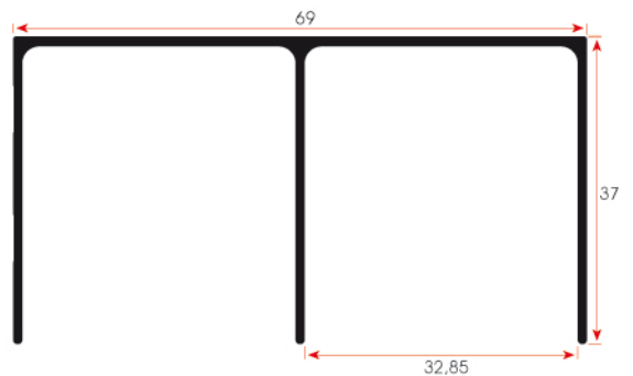
FSM 1025 0,550 kg/m
