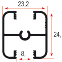
FSM 1003 0,325 kg/m
