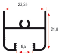
FSM 1004 0,265 kg/m
