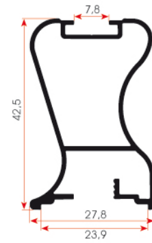
FSM 1041 0,450 kg/m
