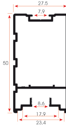
FSM 1007 0,220 kg/m
