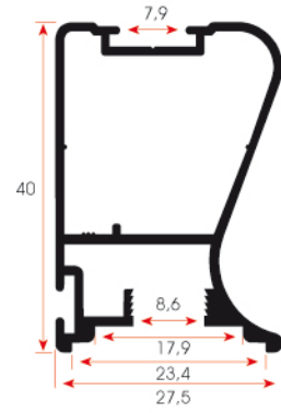
FSM 1022 0,515 kg/m
