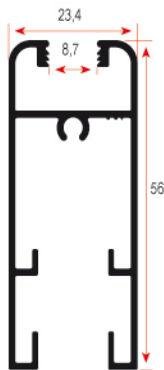
FSM 1021 0,550 kg/m
