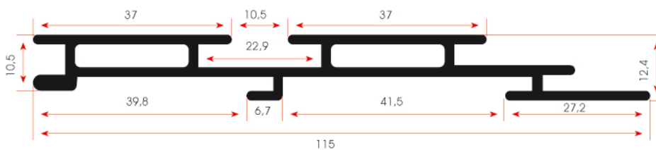
Pano Profili (Birbirine Geçmeli)
