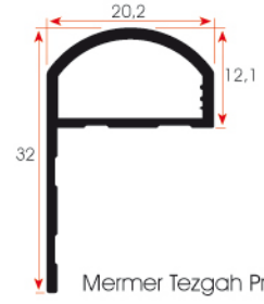
FSM 820 0,250 kg/m
