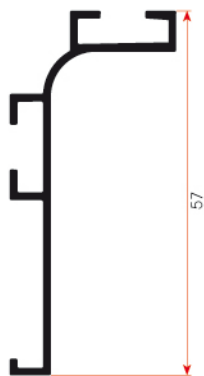
FSM 822 0,362 kg/m
