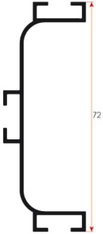
FSM 823 0,655 kg/m
