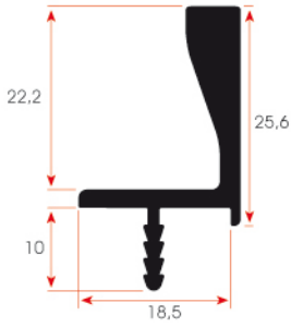
FSM 351 0,340 kg/m
