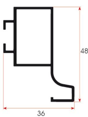
FSM 824 0,526 kg/m
