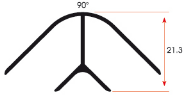
FSM 802 0,245 kg/m
