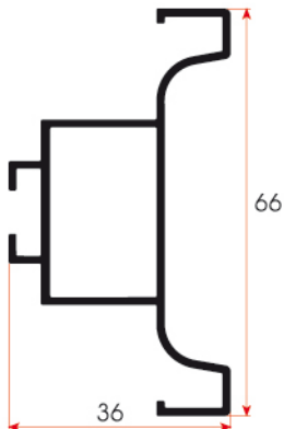
FSM 823 0,655 kg/m
