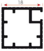
FSM 801 0,250 kg/m
