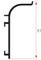
FSM 807 0,319 kg/m
