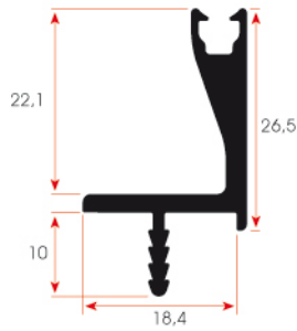
FSM 326 0,381 kg/m
