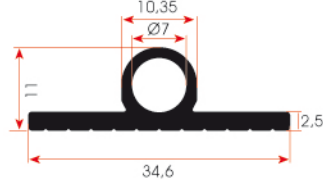
FSM 616 Parçalı Gerğİ Profİlİ
