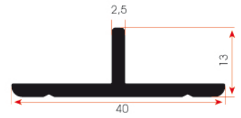
FSM 615 T Gerğİ Profİlİ
