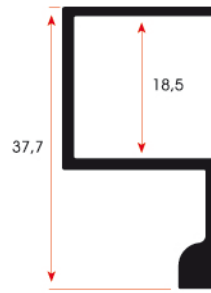
FSM 313 0,335 kg/m
