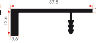
FSM 352 0,345 kg/m
