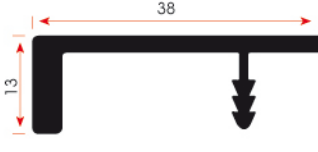
FSM 311 0,405 kg/m
