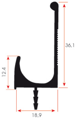
FSM 322 0,415 kg/m
