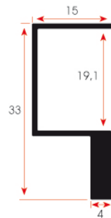
FSM 316 0,262 kg/m
