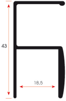
FSM 301 0,380 kg/m
