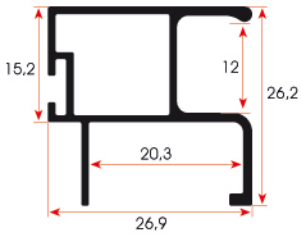
FSM 348 0,317 kg/m
