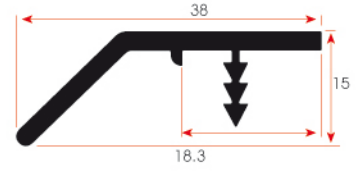
FSM 325 0,375 kg/m
