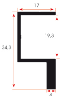
FSM 315 0,347 kg/m
