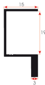
FSM 337 0,210 kg/m
