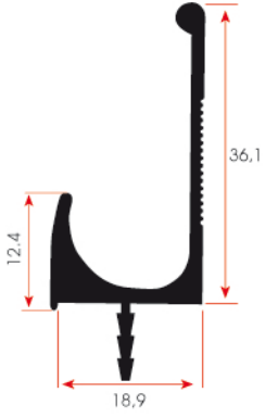
FSM 339 0,595 kg/m
