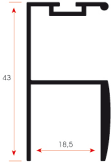
FSM 303 0,410 kg/m
