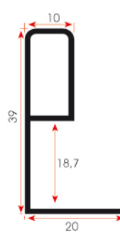
FSM 309 0,285 kg/m
