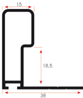
FSM 307 0,454 kg/m
