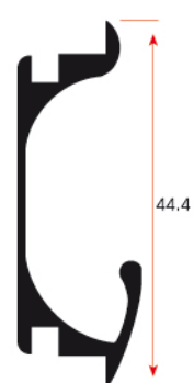
FSM 310 0,373 kg/m
