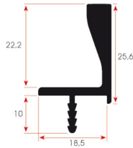
FSM 351 0,340 kg/m
