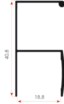
FSM 333 0,260 kg/m
