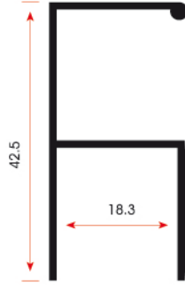
FSM 302 0,305 kg/m
