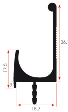
FSM 330 0,460 kg/m
