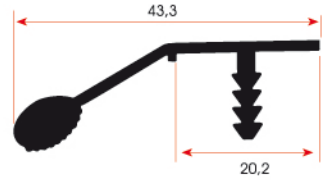
FSM 323 0,395 kg/m
