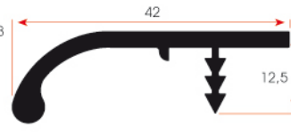
FSM 312 0,405 kg/m
