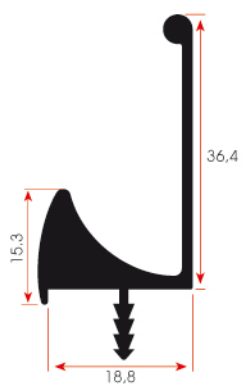
FSM 321 0,515 kg/m
