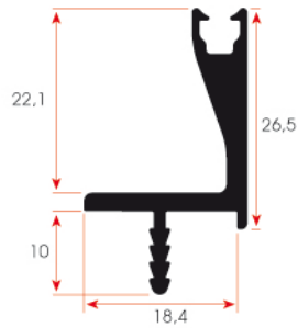
FSM 326 0,381 kg/m
