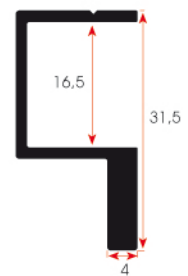
FSM 328 0,330 kg/m
