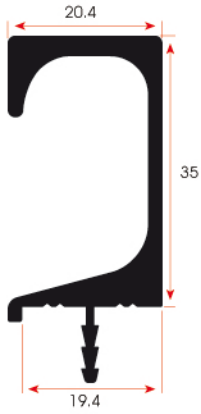
FSM 324 0,207 kg/m
