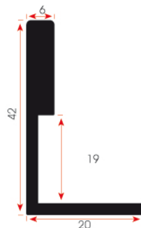
FSM 308 0,630 kg/m
