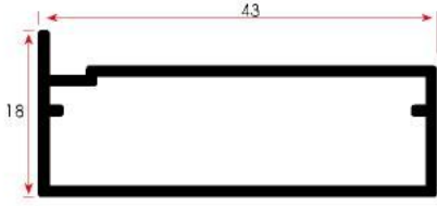
FSM 936 / 0,395 kg/m
