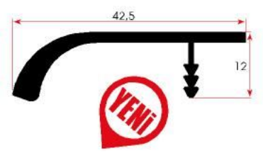
FSM 354 0,365 kg/m
