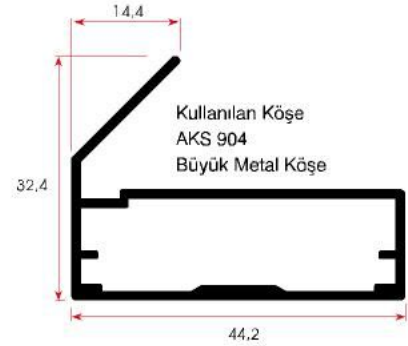
FSM 908 / 0,525 kg/m
