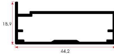
FSM 907 / 0,460 kg/m
