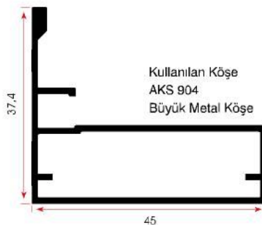
FSM 911 0,520 kg/m
