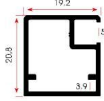
FSM 902 0,282 kg/m
