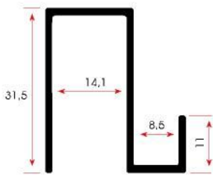
FSM 1019 0,355 kg/m
