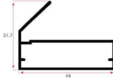
FSM 937 / 0,465 kg/m
