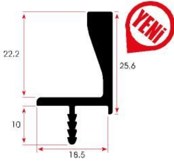
FSM 351 0,340 kg/m
