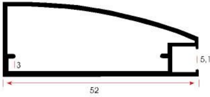
FSM 906 0,468 kg/m
