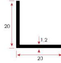
FSM 103 0,128 kg/m
