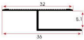
FSM 117 0,139 kg/m
