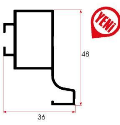
FSM 824 0,526 kg/m
