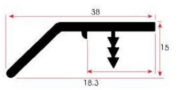
FSM 325 0,375 kg/m
