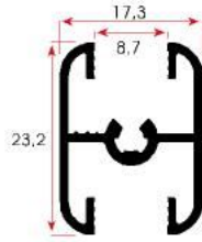
FSM 1035 0,272 kg/m
