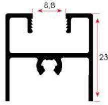
FSM 1013 0,312 kg/m
