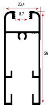
FSM 1021 0,550 kg/m
