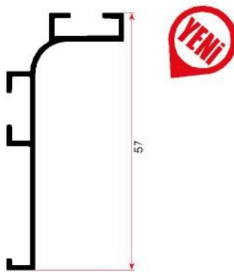
FSM 822 0,362 kg/m
