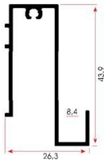
FSM 1020 0,410 kg/m
