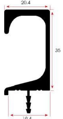
FSM 339 0,595 kg/m
