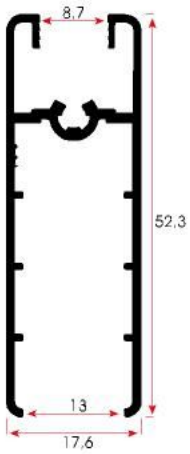
FSM 1007 0,220 kg/m
