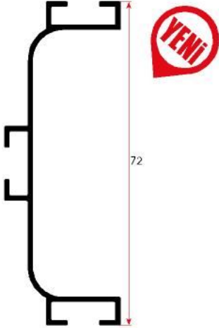
FSM 823 0,655 kg/m
