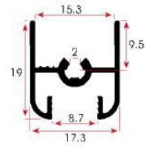
FSM 1036 0,204 kg/m
