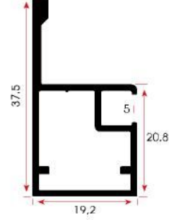
FSM 903 0,380 kg/m
