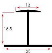
FSM 427
