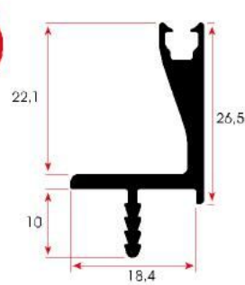
FSM 326 0,381 kg/m
