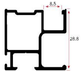
FSM 1017 0,470 kg/m
