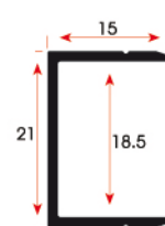
FSM 320 0,160 kg/m
