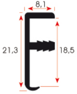
FSM 401 0,149 kg/m
