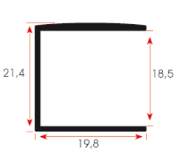
FSM 317 0,205 kg/m
