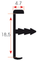
FSM 428 0,141 kg/m
