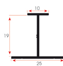
FSM 411 0,160 kg/m
