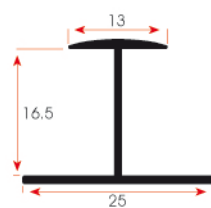
FSM 427 0,160 kg/m
