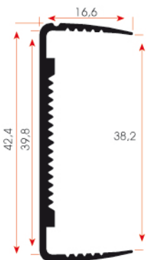
FSM 410 0,295 kg/m
