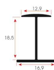
FSM 412 0,136 kg/m
