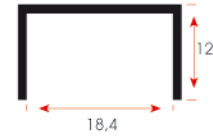
FSM 409 0,127 kg/m
