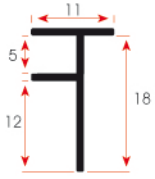
FSM 419 0,097 kg/m
