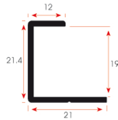
FSM 319 0,169 kg/m
