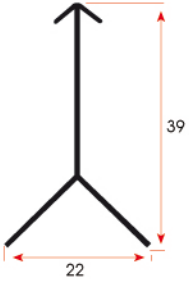
FSM 422 0,225 kg/m
