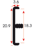
FSM 402 0,111 kg/m
