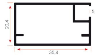
FSM 912 0,366 kg/m
