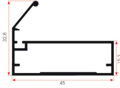
FSM 939 0,475 kg/m
