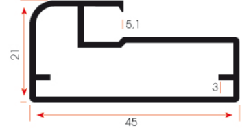
FSM 905 0,452 kg/m
