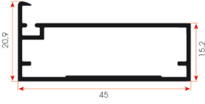
FSM 938 0,425 kg/m
