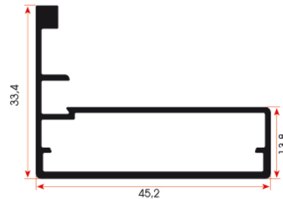
FSM 941 0,525 kg/m
