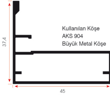
FSM 937 0,465 kg/m
