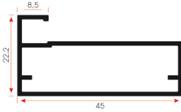
FSM 910 0,444 kg/m
