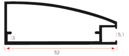
FSM 906 0,468 kg/m
