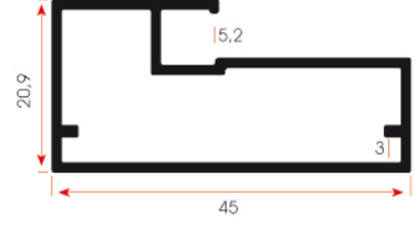
FSM 904 0,430 kg/m
