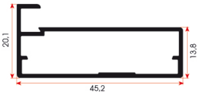
FSM 940 0,415 kg/m
