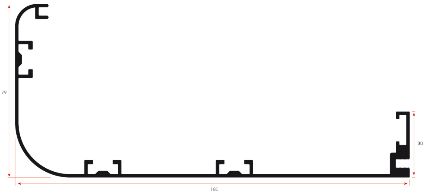
FSM 1506 1,850 kg/m
