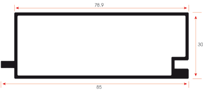
FSM 1503 0,937 kg/m
